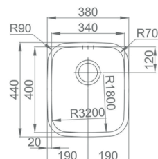
EFR100021000 Fregadero bajo encimera Brasilia pulido 340 x 400
