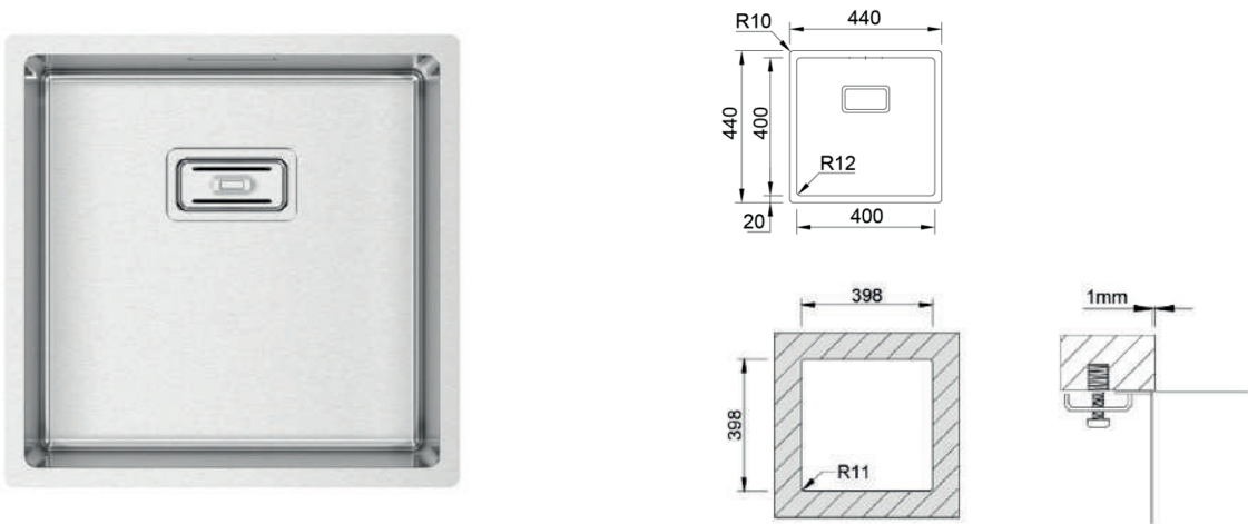
EFR150400000 Fregadero Box lux 40 bajo encimera 400 x 400
