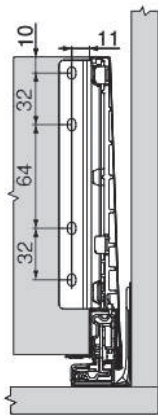
Sección trasera
