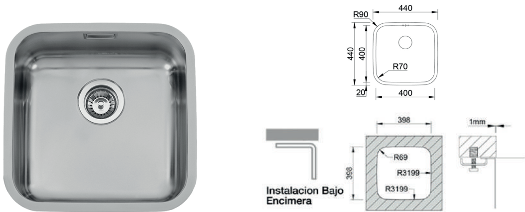
EFR100005000 Fregadero Bahía bajo encimera pulido 400 x 400
