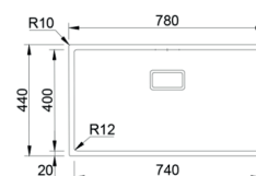
EFR100160000 Fregadero Box lux 74 bajo encimera 740 x 400 V.R.
