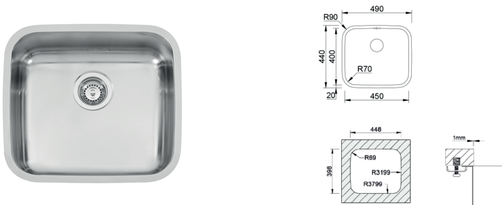
EFR100007000 Fregadero Laguna bajo encimera Pulido 450 x 400
