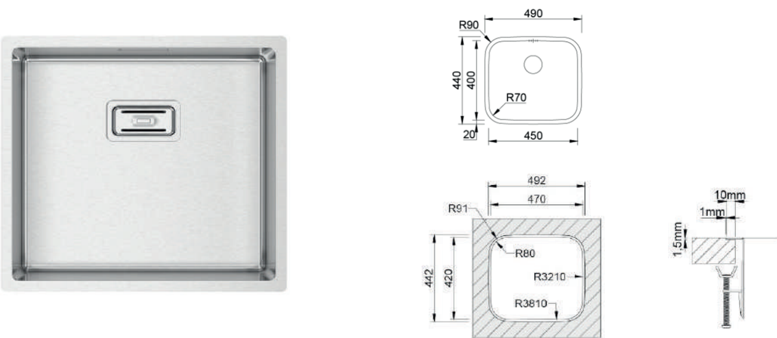
EFR150450000 Fregadero Box lux 45 bajo encimera 450 x 400
