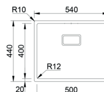
EFR100114010 Fregadero Box lux 50 bajo encimera 500 x 400 V.R.
