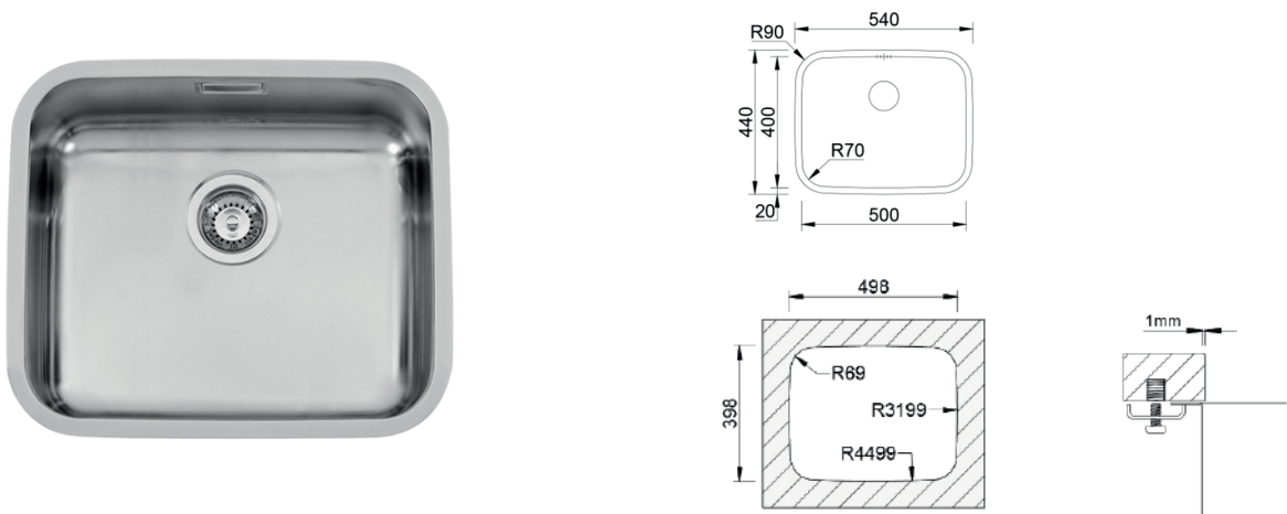
EFR100006000 Fregadero Belem bajo encimera pulido 500 x 400
