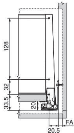
Dimensiones instalación
